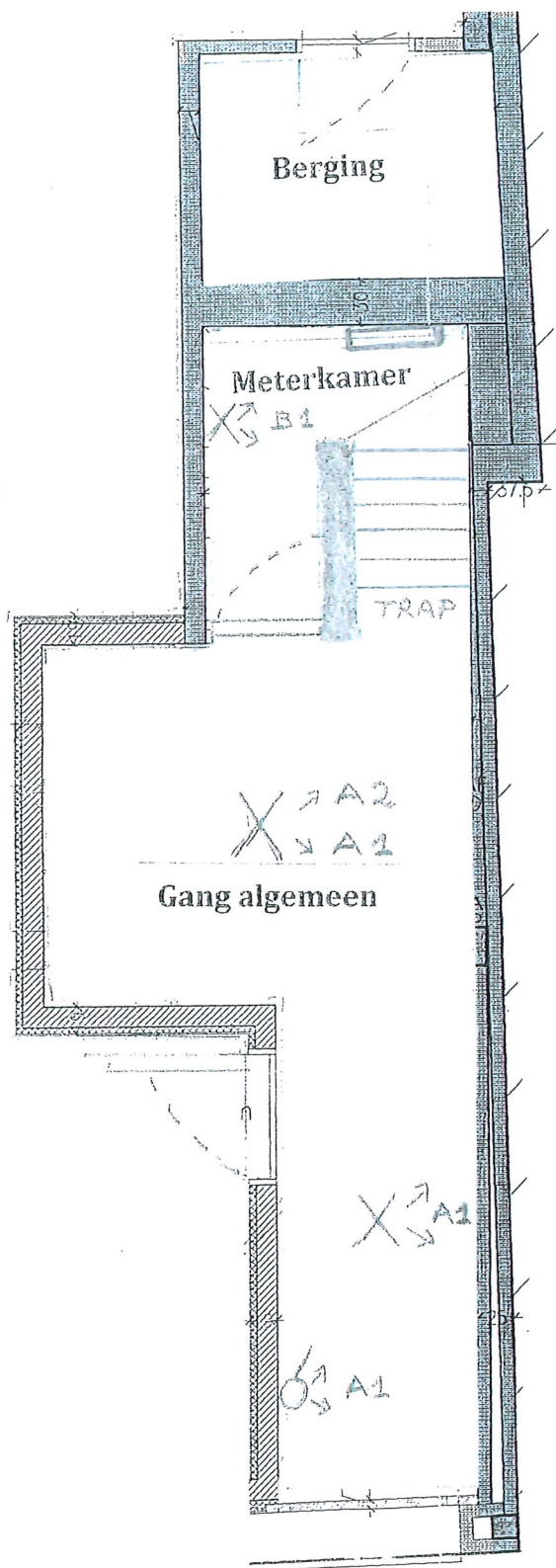
GRONDPLAN BENEDEN
