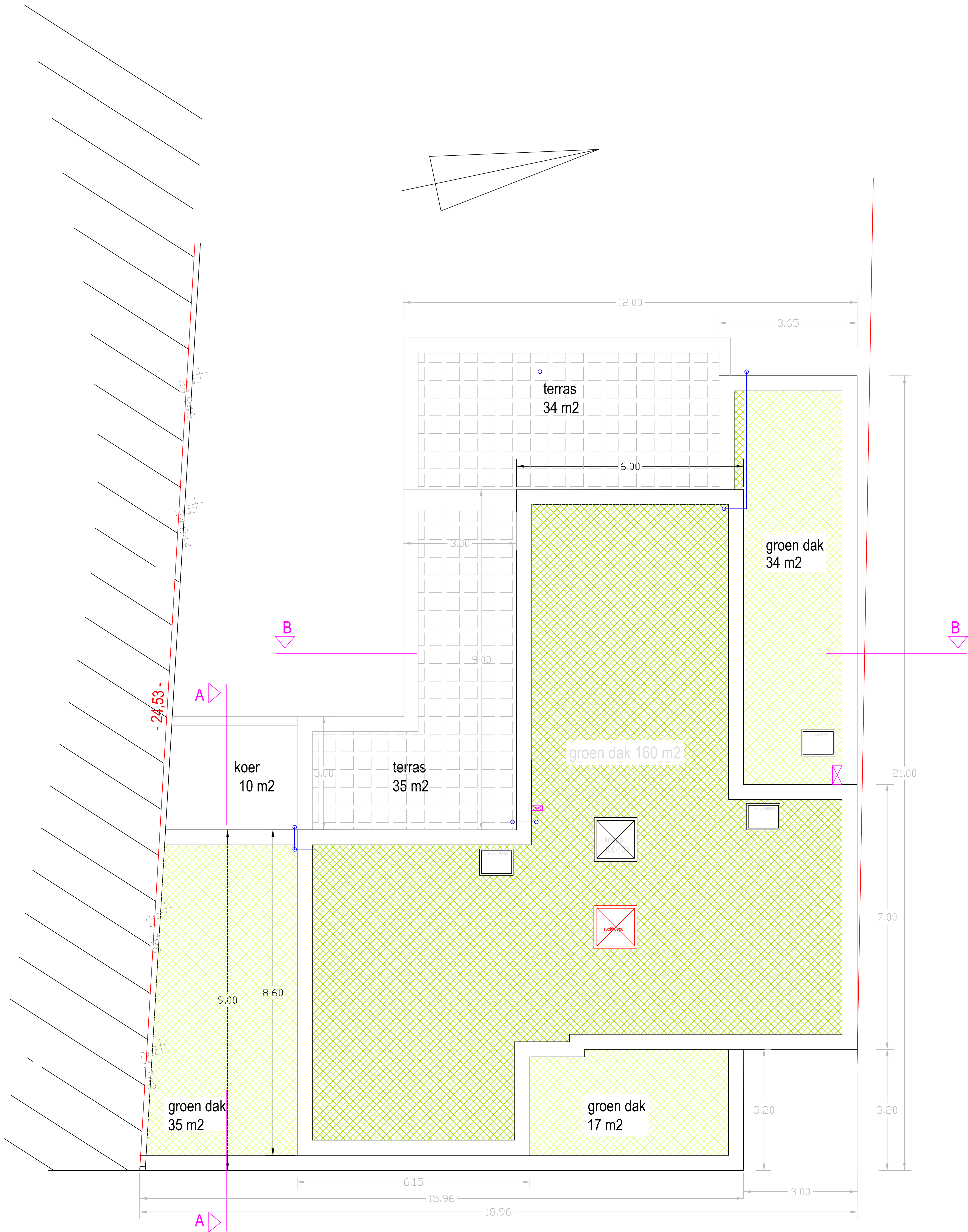
DAK schaal 1/50
