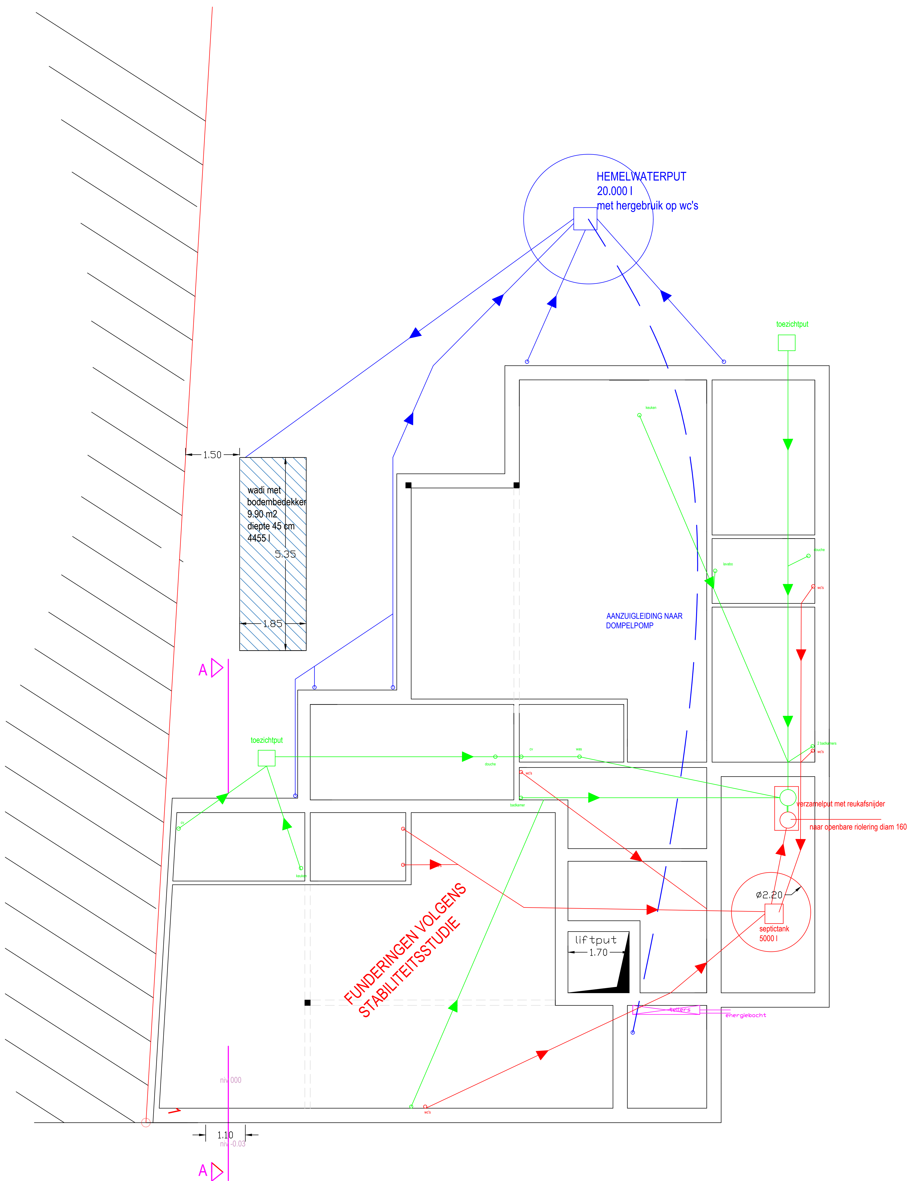
RIOLERINGSPLAN schaal 1/50
